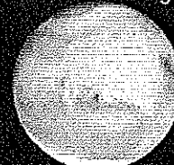
Mars
